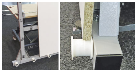
Für Plattenverarbeiter gibt es den Hubtisch auch mit seitlich montiertem Schwenkrahmen
